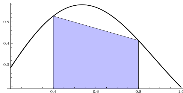
Slika 2: Trapez ispod funkcije e^{\sqrt{x}} \sin x \cos^4 x na [0.4, 0.8] .
