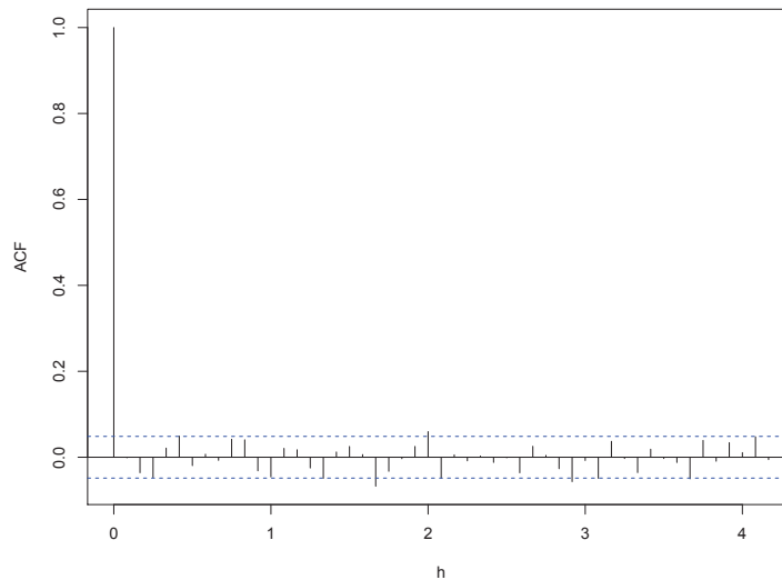
Slika 4.15: Procijenjena autokorelacijska funkcija reziduala modela (4.3).
