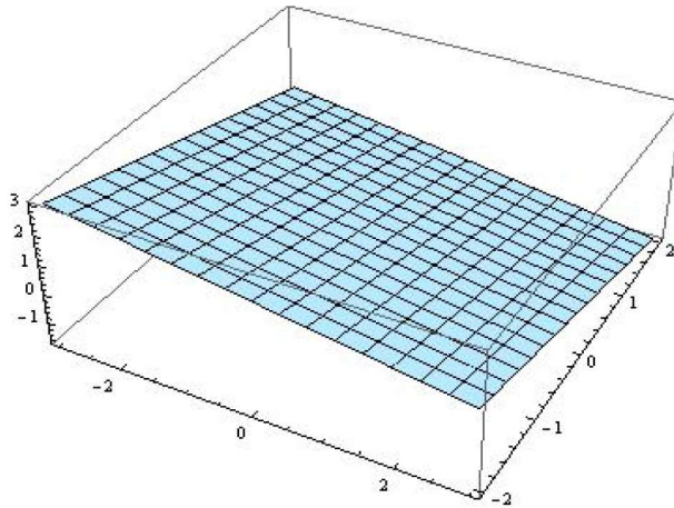
Slika 2: Hiperravnina H u \mathbb{R}^3 : x_1 + 2x_2 + 3x_3 = 2 , tj. a = (1, 2, 3) , x = (x_1, x_2, x_3) , \beta = 2
