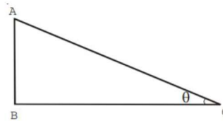
SLIKA 33. Pravokutan trokut
