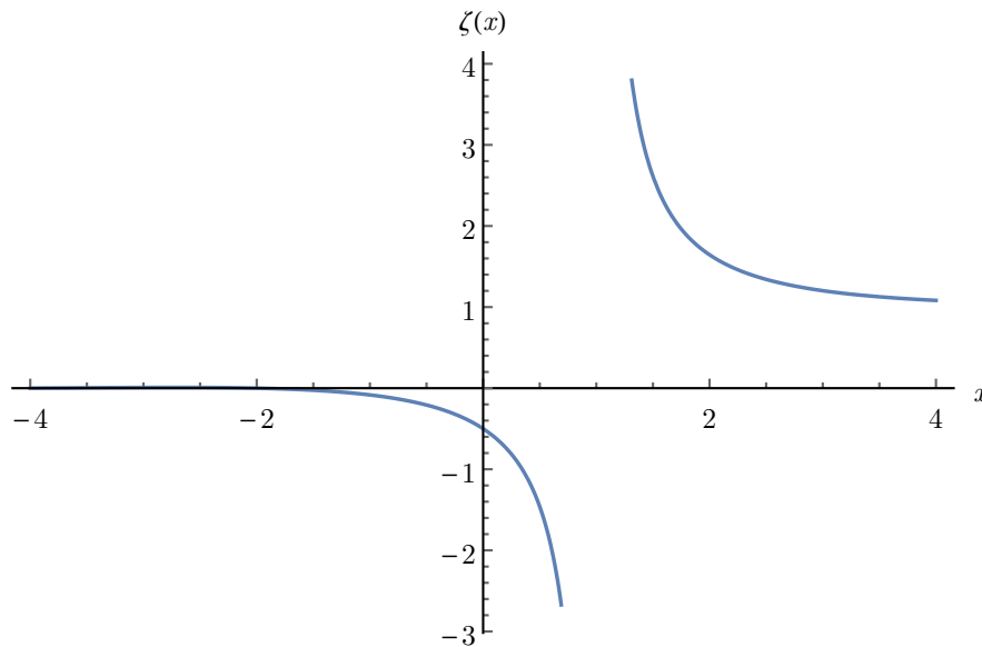
Slika 3.2: Graf Riemannove zeta funkcije
