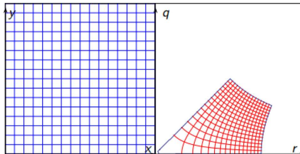
Slika 10. Konformno preslikavanje kvadrata funkcijom w(z) = \sqrt{z}
