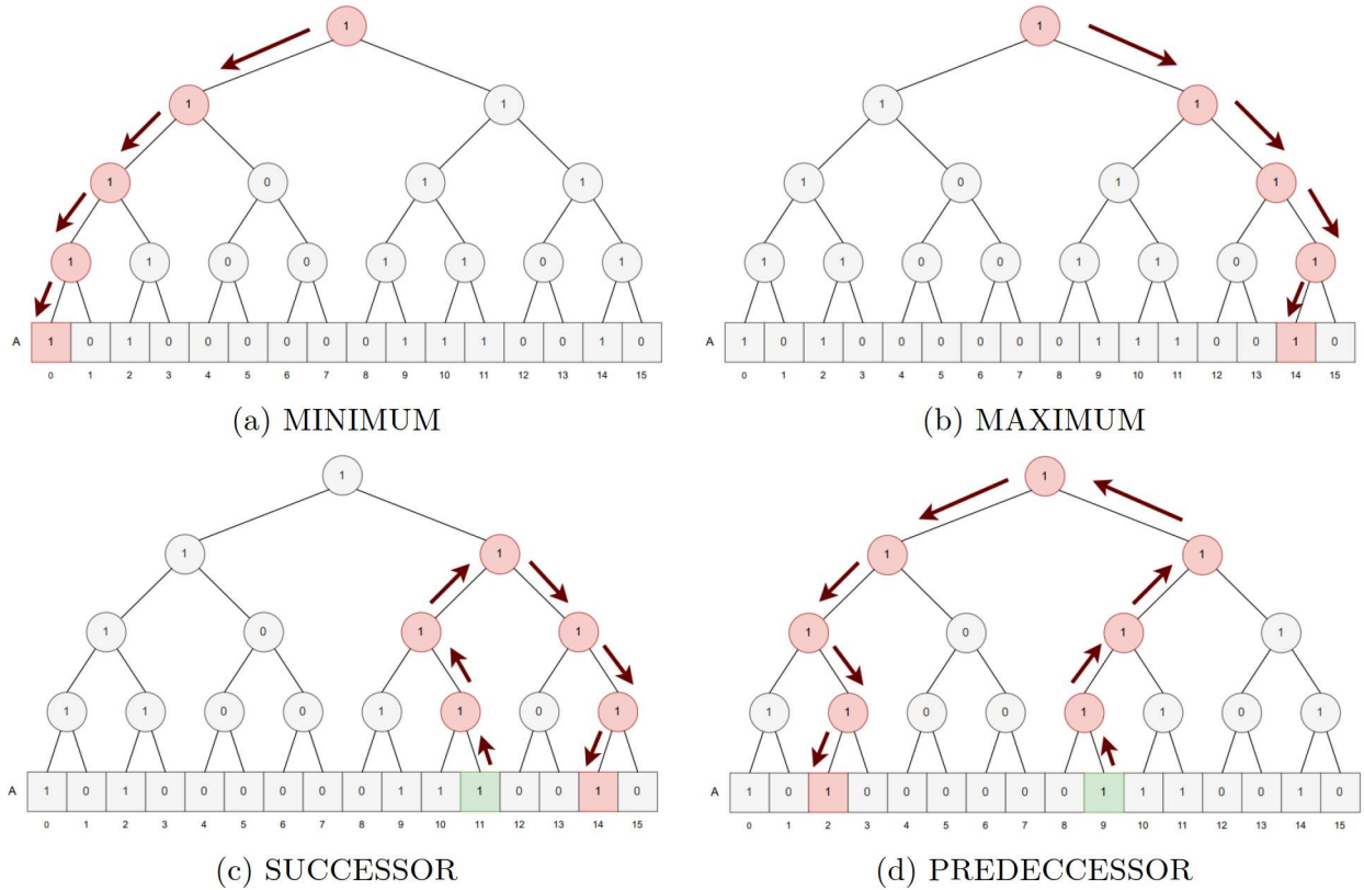
Slika 3: Strjelice prikazuju putanja za pronalazak: (a) minimuma skupa \{0, 2, 9, 10, 11, 14\} . (b) maksimuma skupa \{0, 2, 9, 10, 11, 14\} . (c) sljedbenika broja 11 iz skupa \{0, 2, 9, 10, 11, 14\} . (d) prethodnika broja 9 iz skupa \{0, 2, 9, 10, 11, 14\} .
