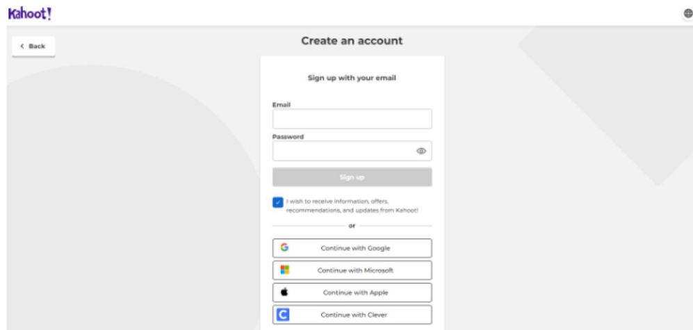
Slika 20: Izrada računa
