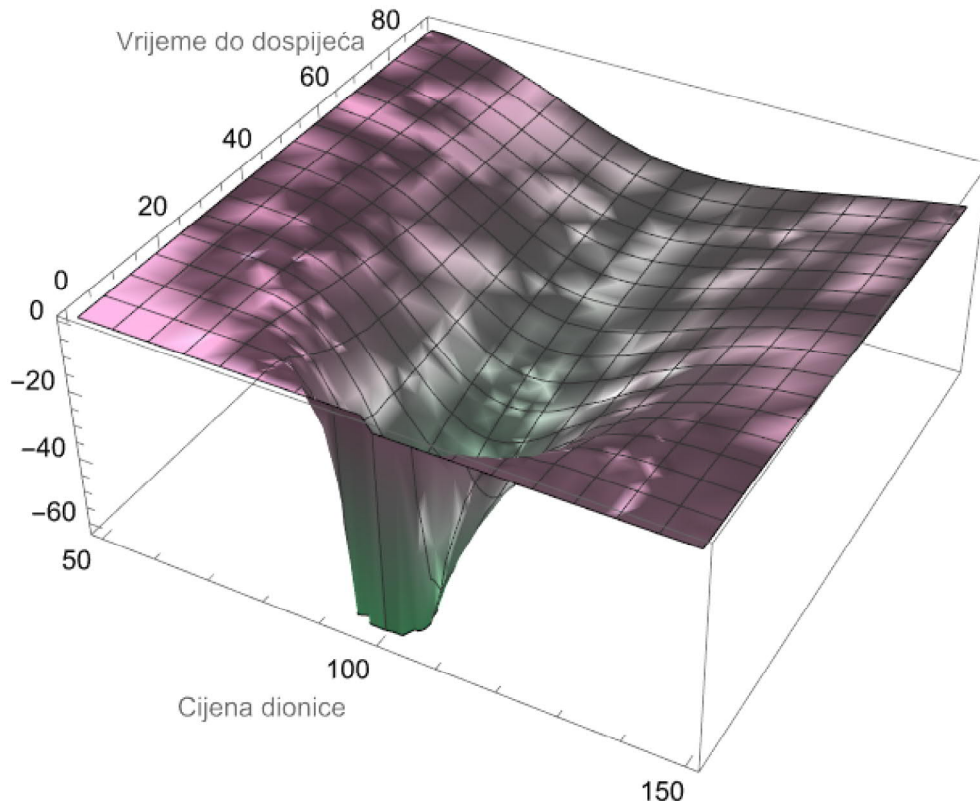
Slika 14: Vrijednost thete call opcije s obzirom na cijenu dionice i vrijeme do dospjeća za K = 100
