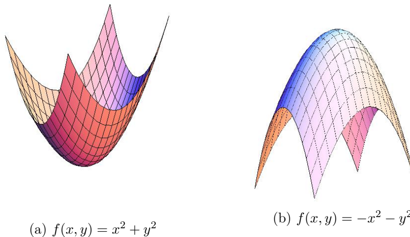
Slika 2.6: Funkcije f(x, y) = x^2 + y^2 i f(x, y) = -x^2 - y^2 (eliptički paraboloid)
