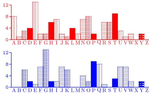
Slika 3.4: Usporedba učestalosti otvorenog teksta i šifriranog teksta za svako šesto slovo primjera Vigenereove šifre, počevši s prvim slovom
