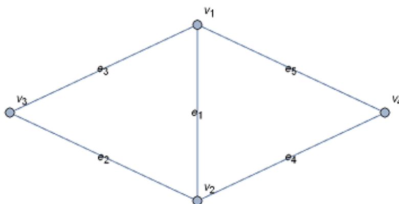
Slika 1: Graf G
