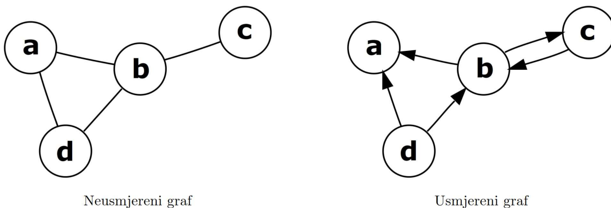
Slika 1: Primjeri neusmjerenog i usmjerenog grafa sa 4 vrha.
