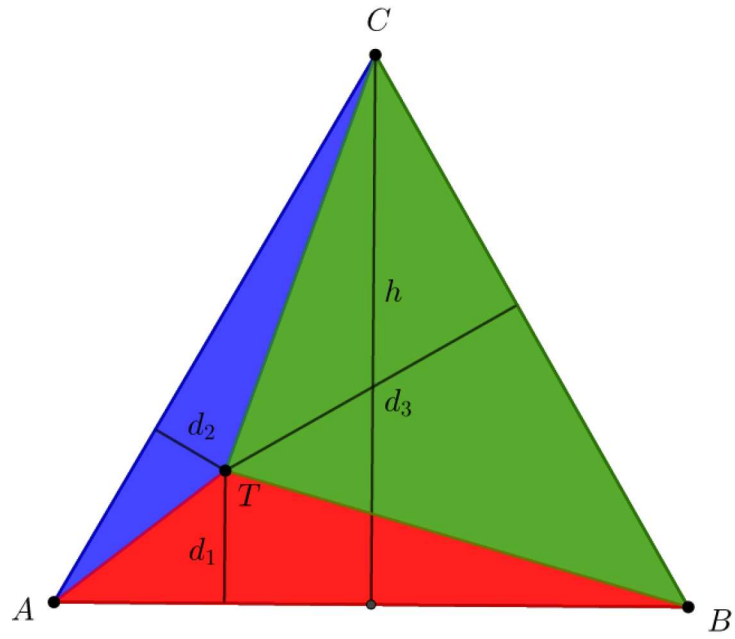
Slika 3: Dokaz pomoću površina
