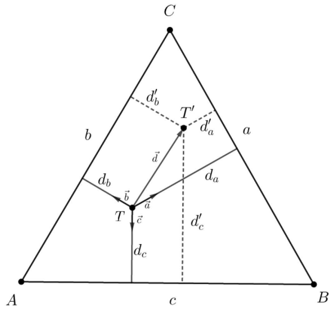
Slika 6: Dokaz pomoću vektora
