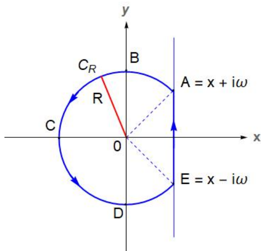
Slika 3: Bromwicheva kontura
