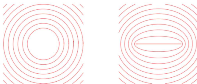
Slika 14. Joukowski preslikavanje
