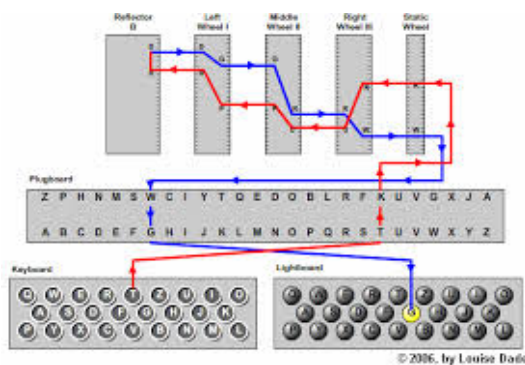
Slika 13: Struktura Enigme
