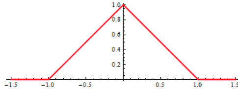
Slika 3: Funkcija gustoće slučajne varijable X
