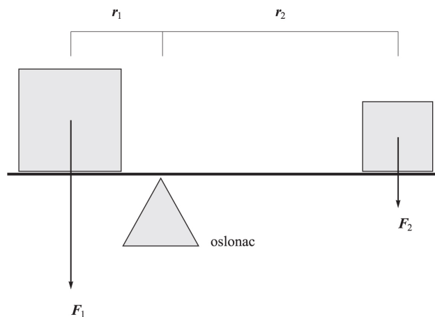
Slika 20: Zakon poluge
