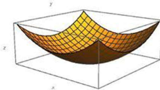
Slika 5: Graf funkcije f(x, y) = x^2 + y^2 koja postiže lokalni minimum u točki (0, 0)
