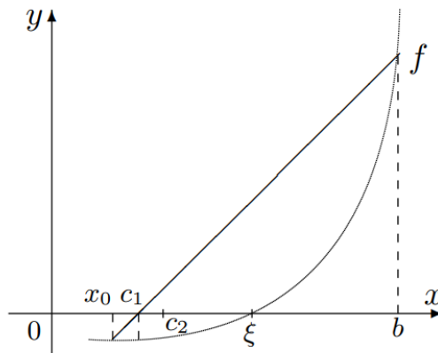
Slika 3: Regula falsi
