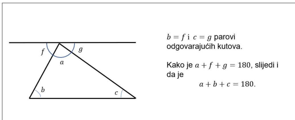
Slika 4.1: Zbroj kutova u trokutu
