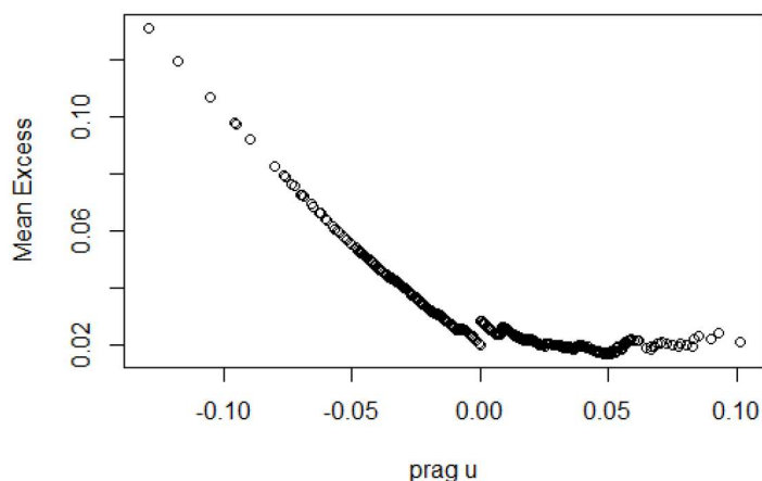
Slika 9: ME funkcija log-povrata Saponije
