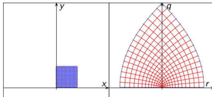
Slika 8. Konformno preslikavanje kvadrata funkcijom w(z) = z^2
