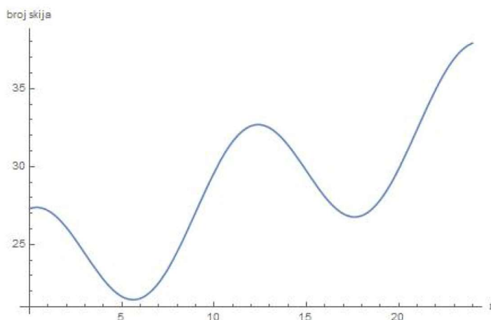
Slika 22: Graf funkcije (14)
