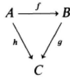
Slika 1: Komutativni dijagram, Izvor ([9])
