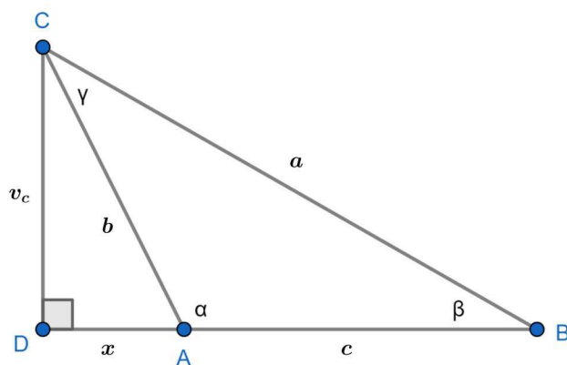
Slika 3.5: \alpha > 90^\circ .
