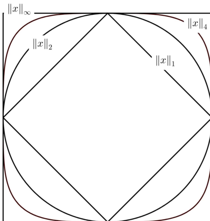
Slika 2.2: Jedinična sfera
