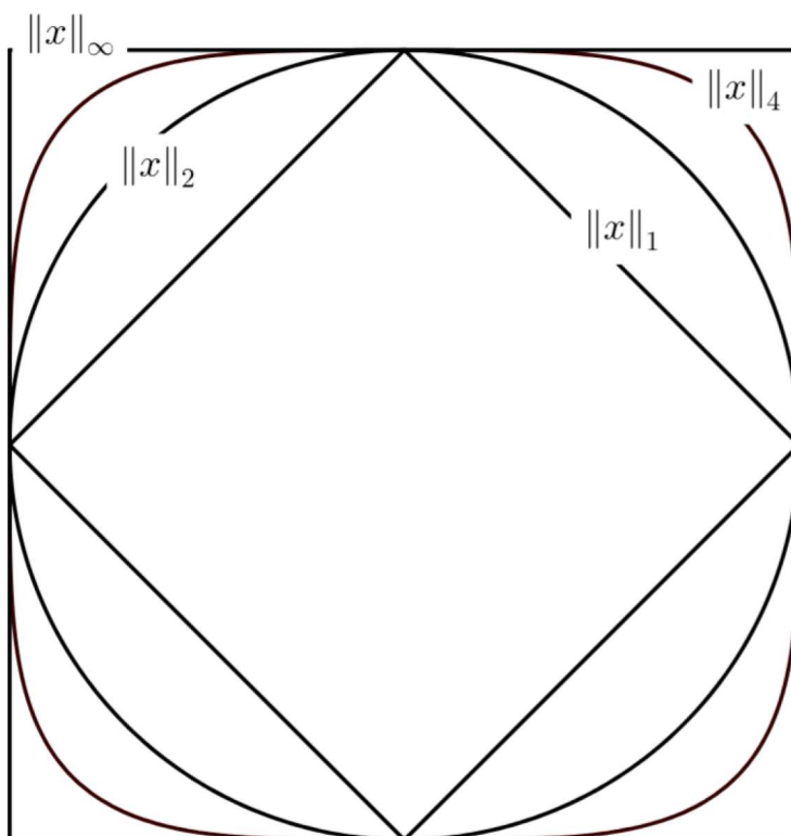
Slika 2.2: Jedinična sfera
